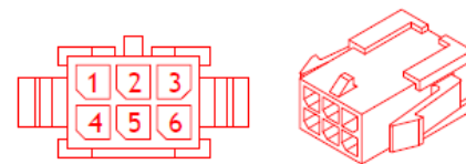
Molex 43020-0600
