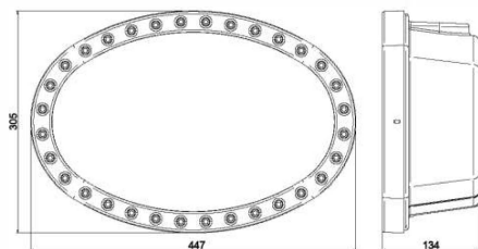
Figure 4: Ellipse Mini model
